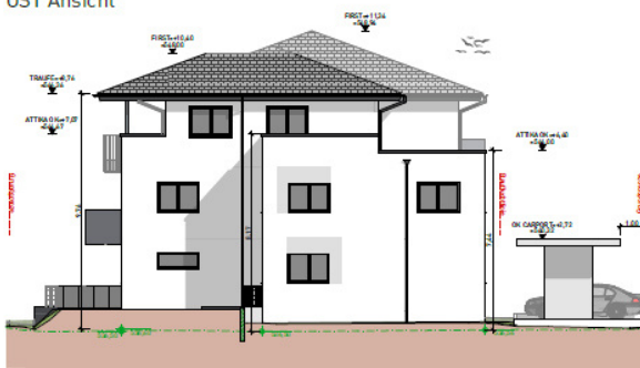
OST Ansicht
